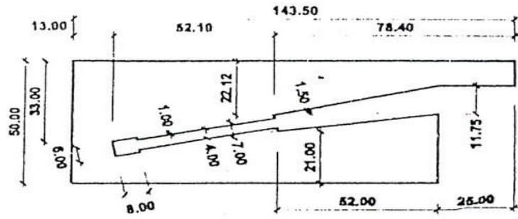
Detalhe dos braços Escala: 1/20
