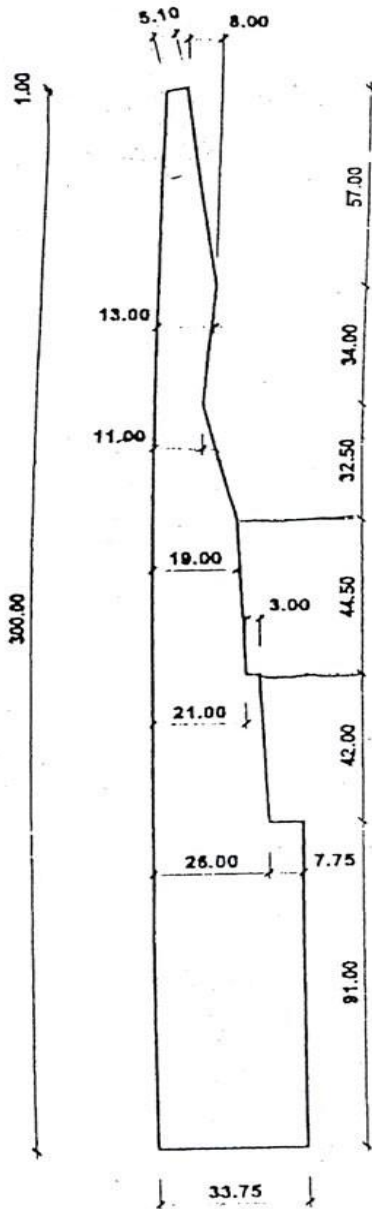
Detalhe do tronco Escala: 1/20
