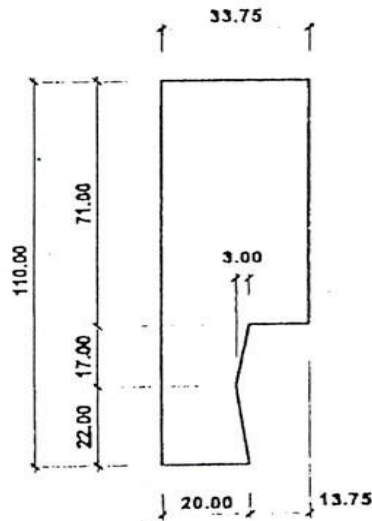
Detalhe da cabeça Escala: 1/20
